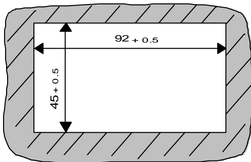
Découpe d'encastrement
